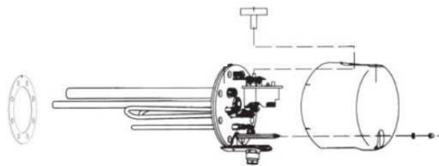
TRF Габаритный чертеж
